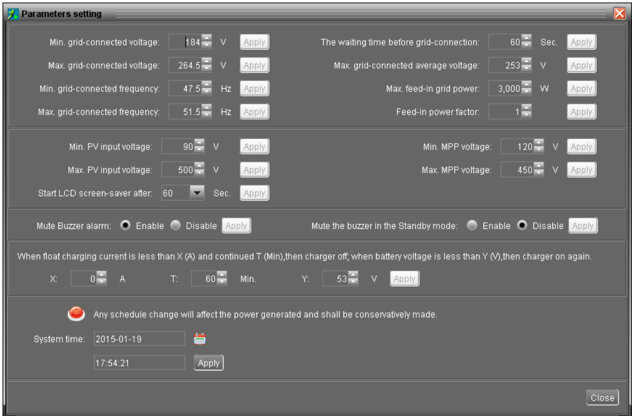
Diagram 4-11B (Grid-Tie mode)
